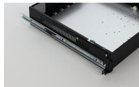
Zdemontuj prowadnicę
