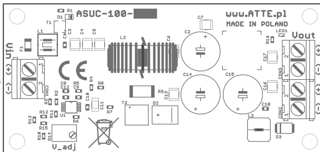
Rys. 1. Widok urządzeń ASUC-100-480-OF oraz ASUC-100-AD0-OF
