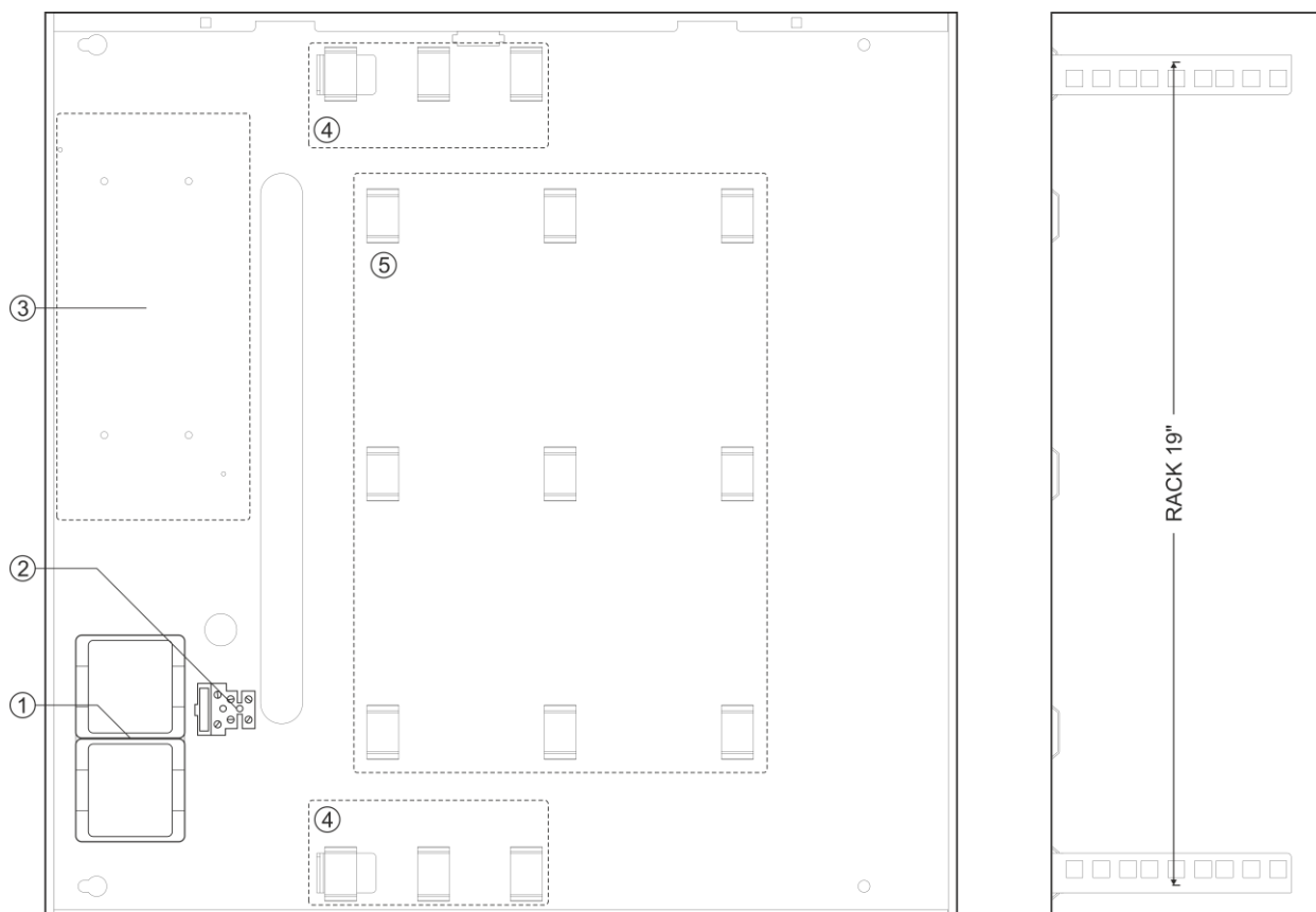
Rys.1 Widok obudowy
