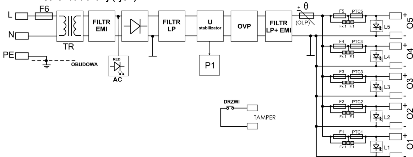
Rys.1. Schemat blokowy zasilacza.
