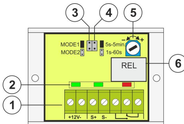
Rys. 1. Widok modułu.
