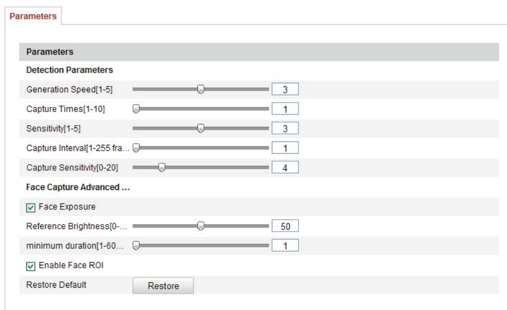
Figure 5-73 Konfiguracja zaawansowana
