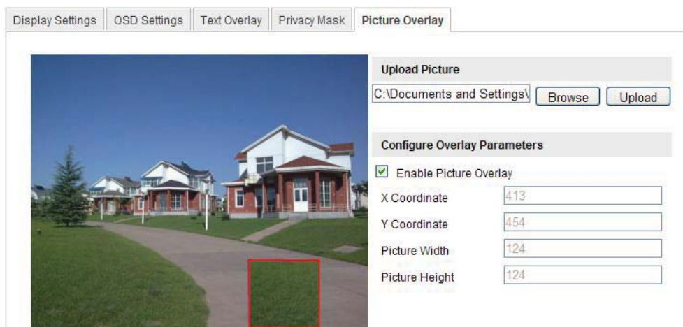
Figure 5-43 Nakładanie obrazów
