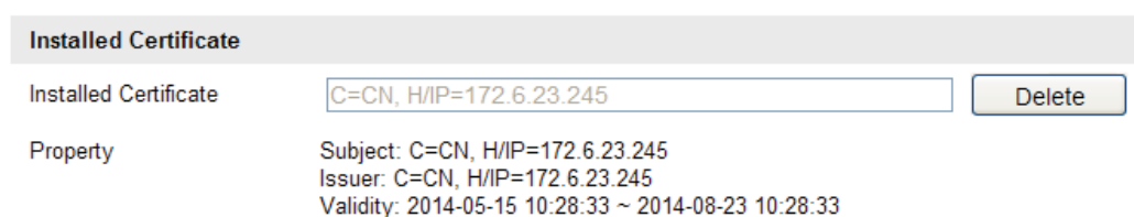
Figure 5-28 Zainstalowany certyfikat
