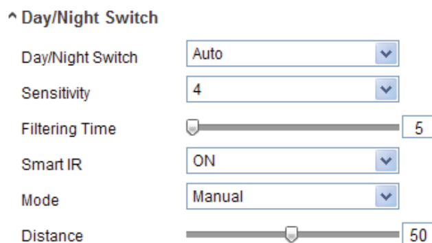
Figure 5-35 Przełączanie Dzień/Noc
