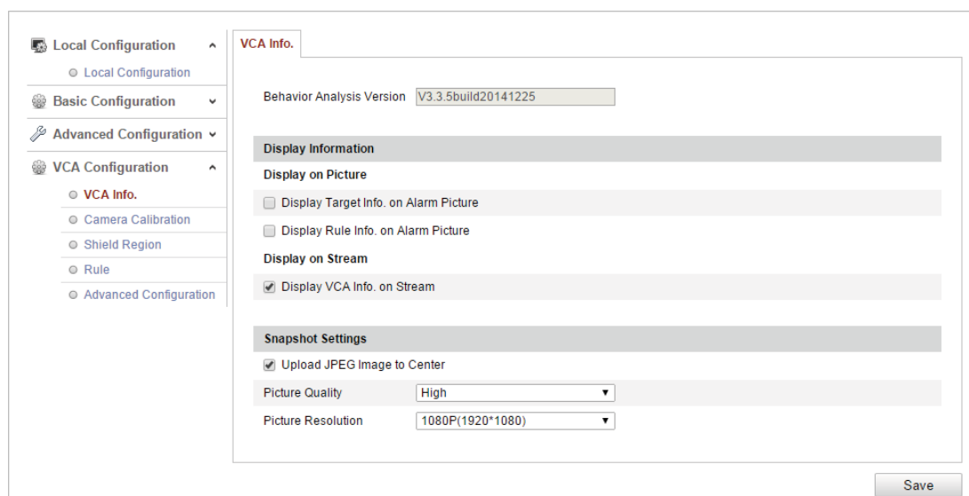
Figure 5-68 Analiza zachowań
