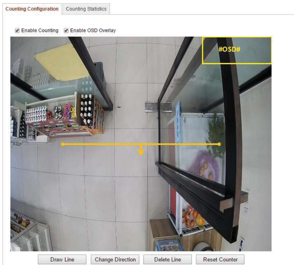
Figure 7-1 Konfiguracja liczenia
