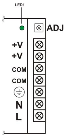
Rysunek 1. Opis złącz zasilacza.
