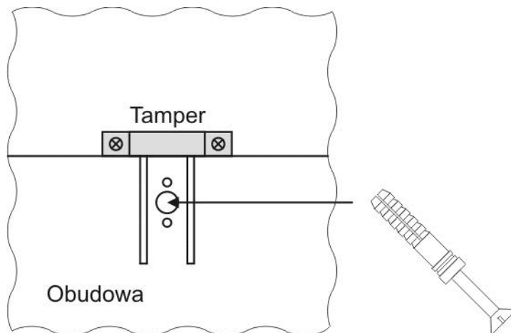
Rys. 4. Montaż uchwyту tampera antysabotażowego.
