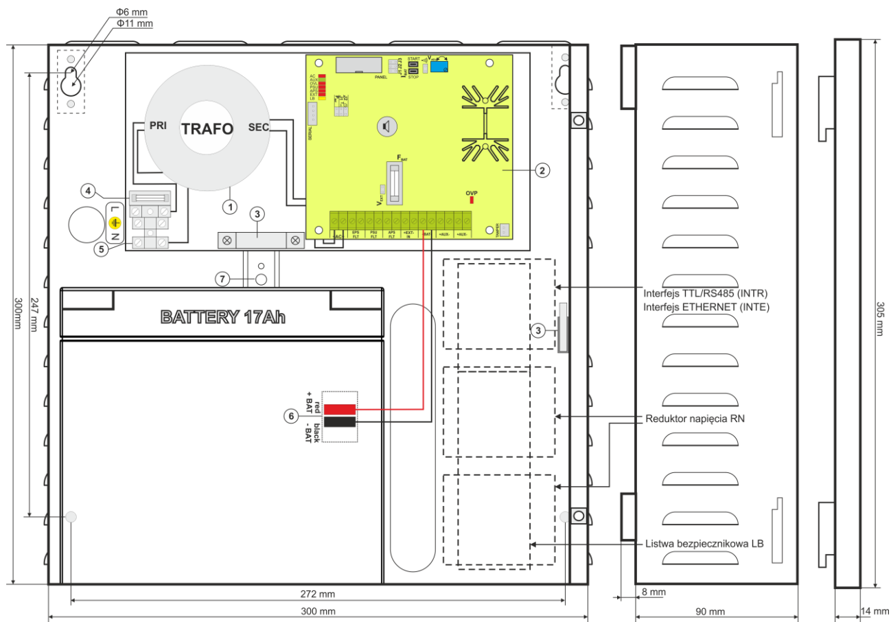
Rys.3. Widok zasilacza.
