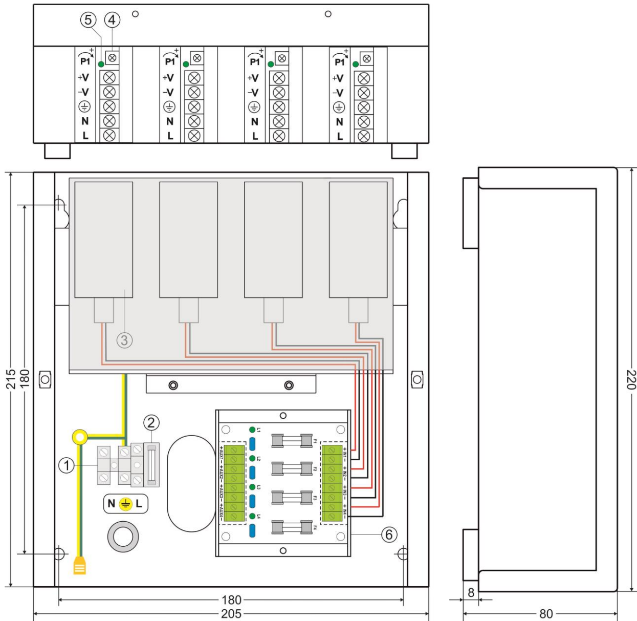
Rys.3. Widok zasilacza.
