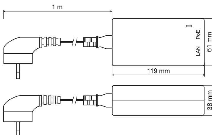
Rys.1. Widok mechaniczny zasilacza.
