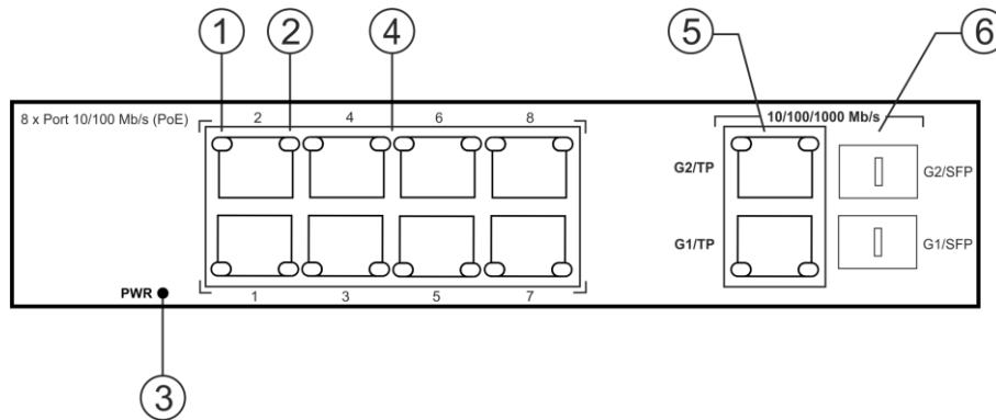
Rys.5. Widok Switch'a.
