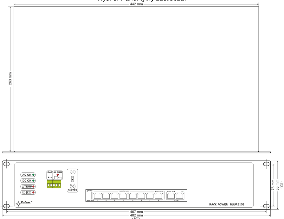
Rys.4. Widok zasilacza.
