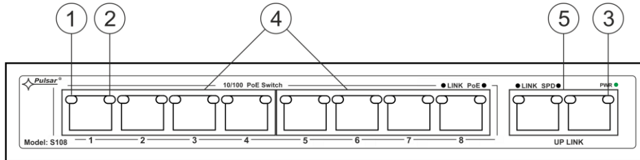
Rys.5. Widok Switch'a.
