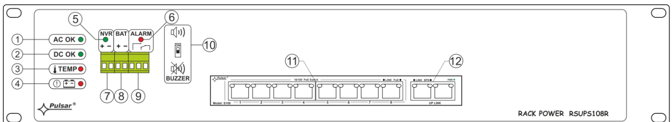
Rys. 3. Panel czołowy zasilacza.
