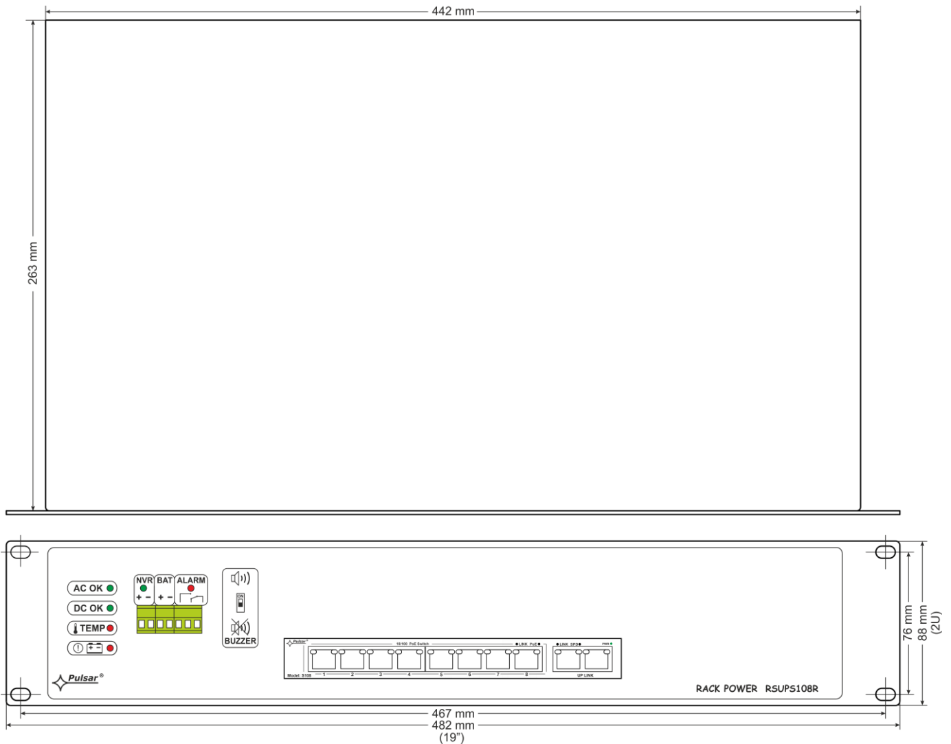
Rys.5. Widok zasilacza.
