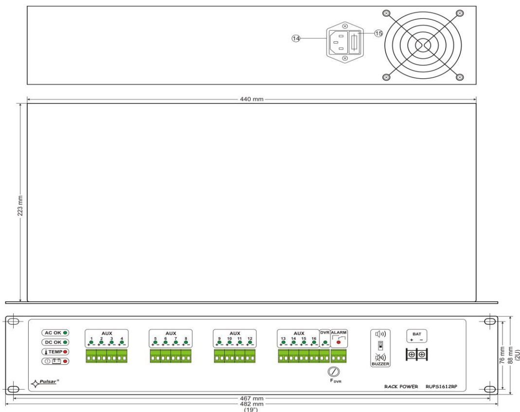
Rys.3. Widok zasilacza.
