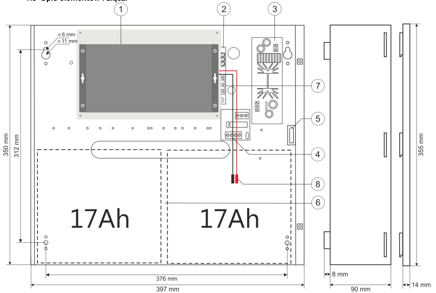
Rys. 2. Widok obudowy.
