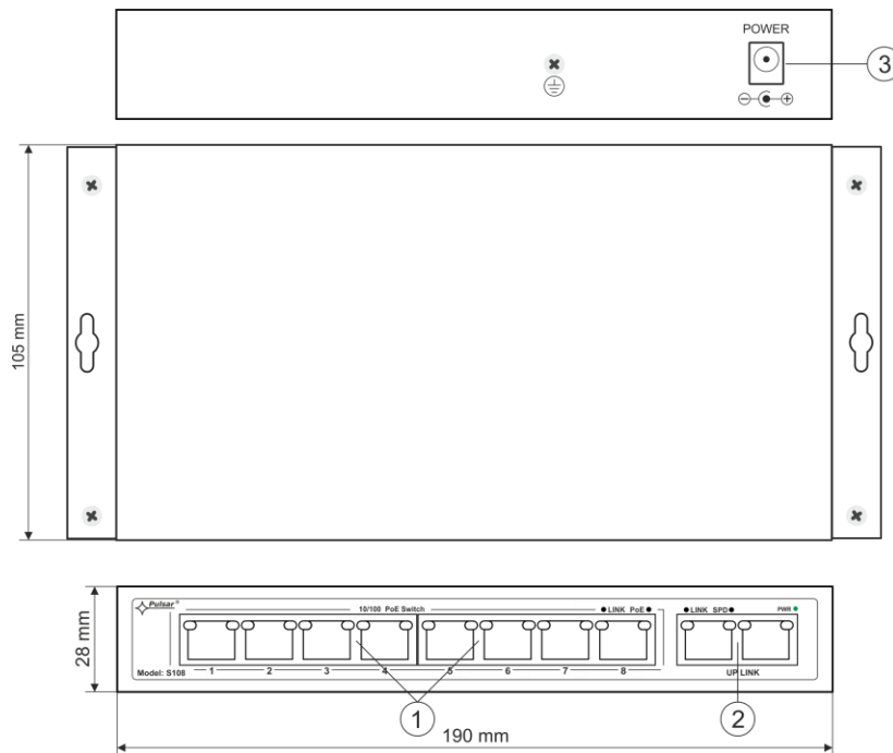
Rys. 3. Widok switch'a.
