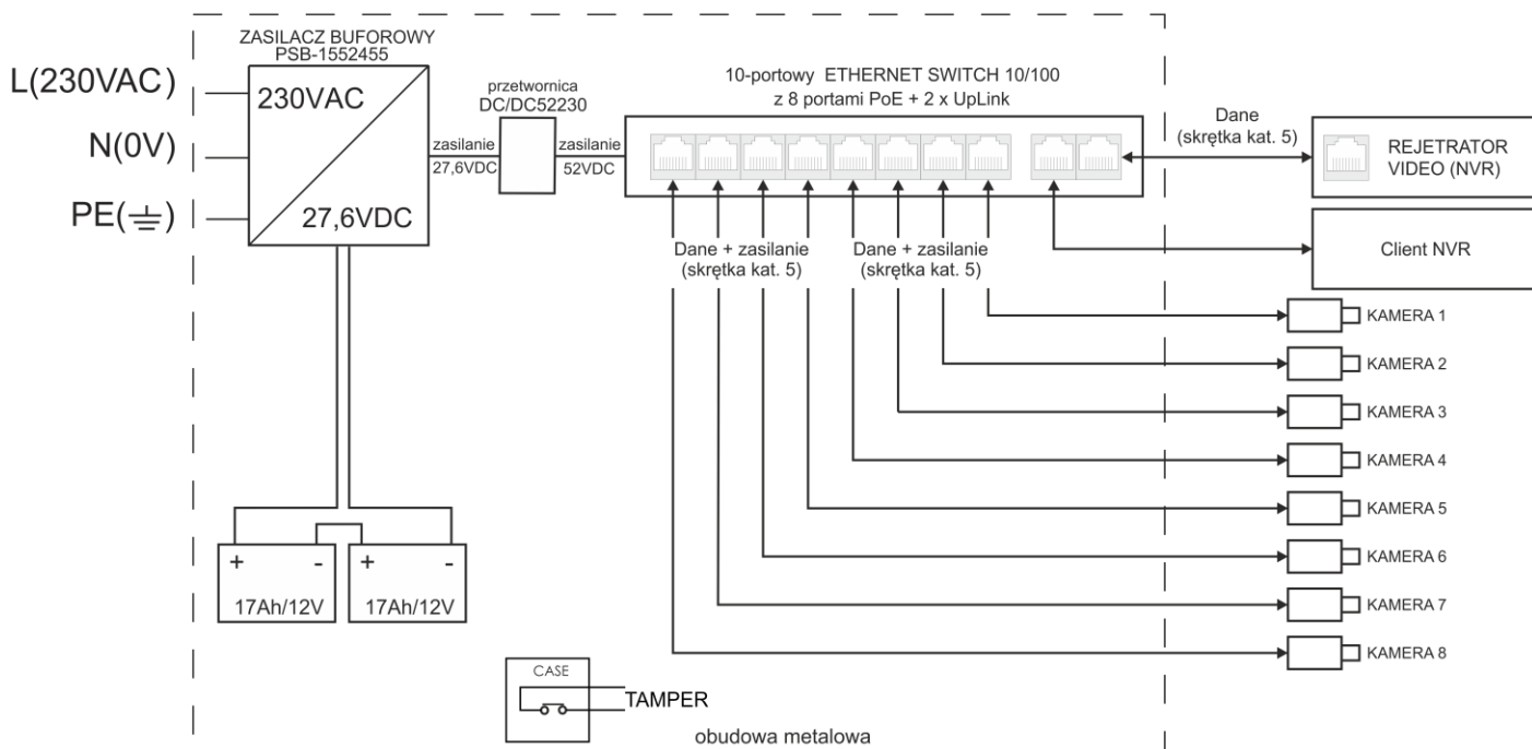
Rys. 1. Schemat blokowy.
