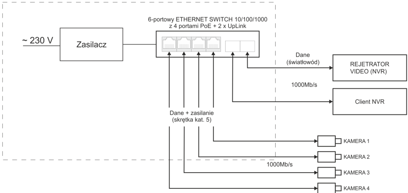
Rys. 1. Schemat blokowy.
